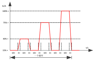
IEC 60269-6:2010 电流循环测试波形
