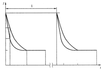
GBT 31465.1-2015 电流循环冲击脉冲
