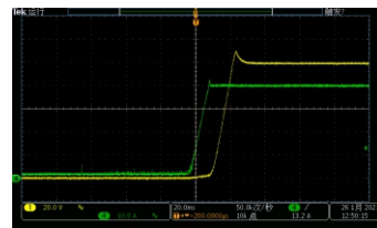
CC优先 (高速建立电流, 电压超调)
