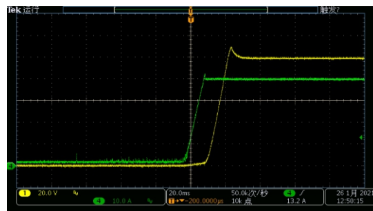
cc优先（高速建立电流，电压超调）
