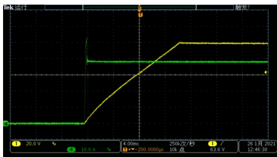
cv优先（高速建立电压，电流超调）
