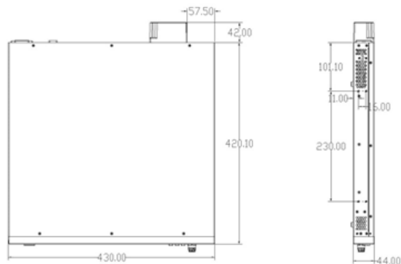
1200W、1500W、1800W机型尺寸：
