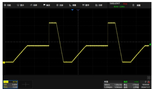
序列测试输出波形
