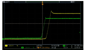
CC优先（高速建立电流，电压超调）
