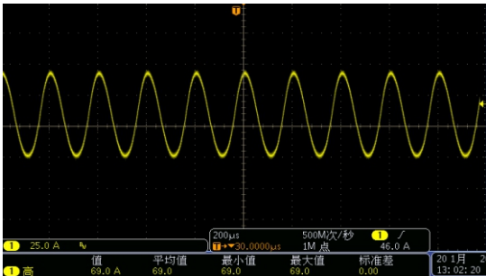
5 kHz正弦波
